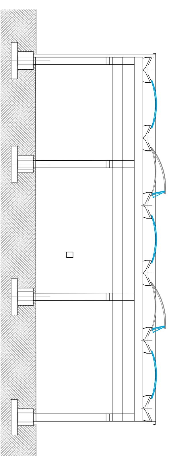
SEZIONE B-B
